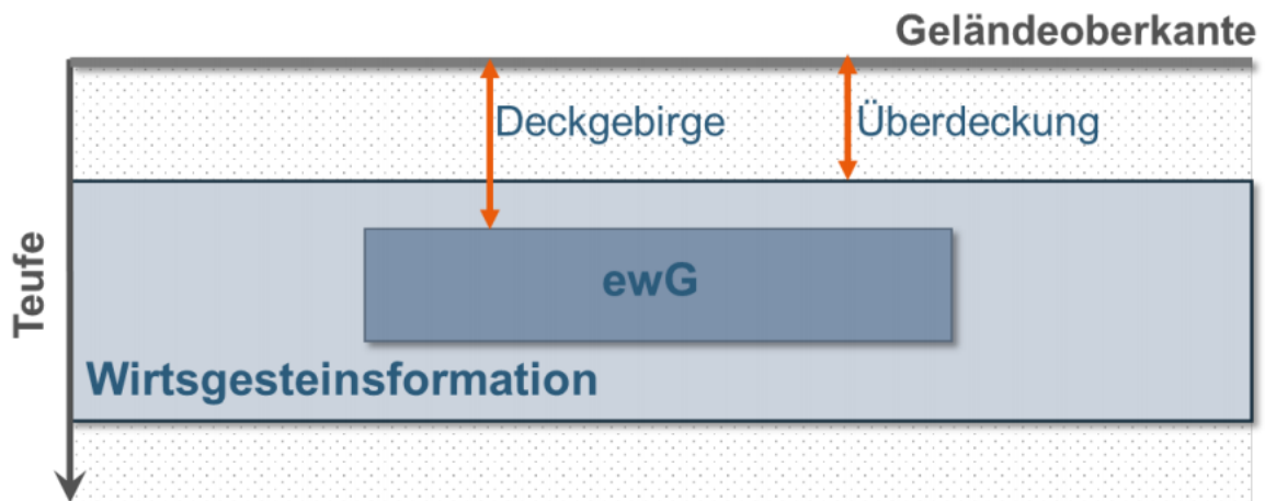
Abbildung 1: Schematische Darstellung der Ausdehnung des Deckgebirges und der Überdeckung (ewG = einchlusswirksamer Gebirgsbereich)
