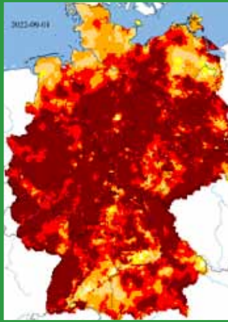
Dürrekarte des Hemholtz Zentrums: Am 1. September 2022 galt für fast ganz Deutschland die höchste Stufe: außergewöhnliche Dürre
